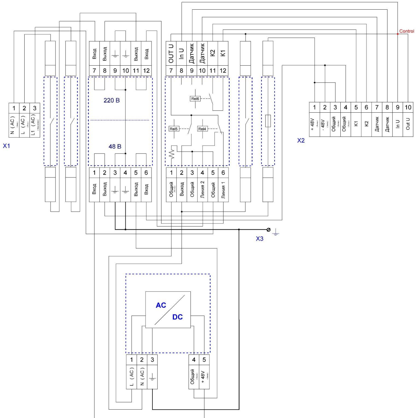
Рисунок 5. Схема структурно-принципиальная.
