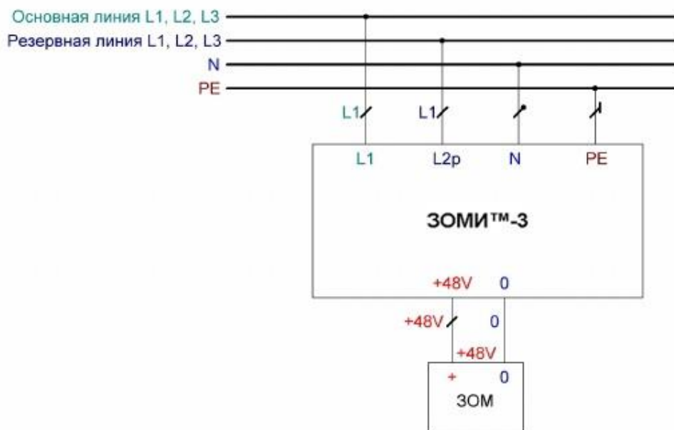
Рисунок 4. Однолинейная схема.
