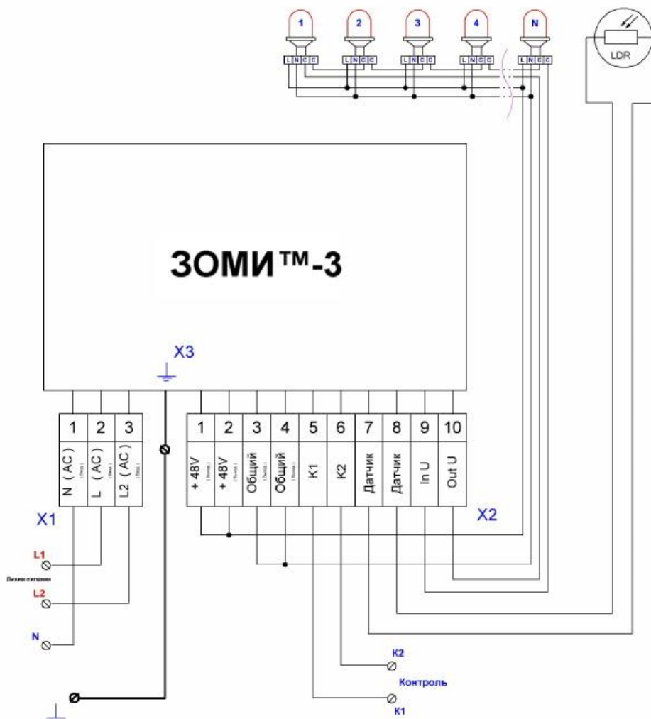
Рисунок 2. Схема подключения.
